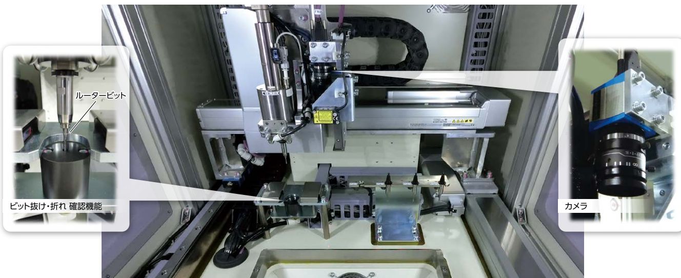
正面から見た装置内部
